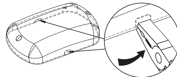
Рисунок 3 — Расположение выламываемых вставок в корпусе светильника СА-7006Д
