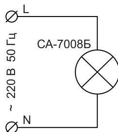
Рисунок 6 — Схема подключения светильника СА-7008Б
