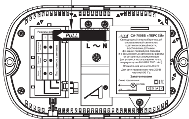
Рисунок 5 — Местоположение транспортировочной плёнки-изолятора
