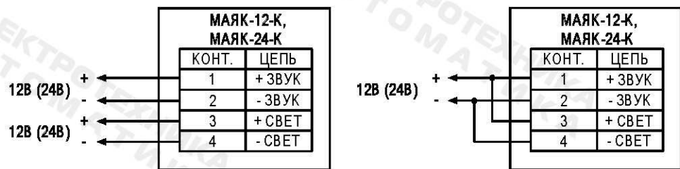
Рис.1. Схема подключения.
