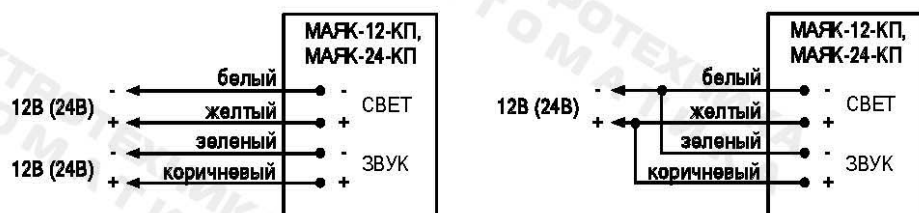
Рис.1. Схемы подключения.
